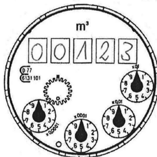
Muster eines Zählwerks eines Wasserzählers
