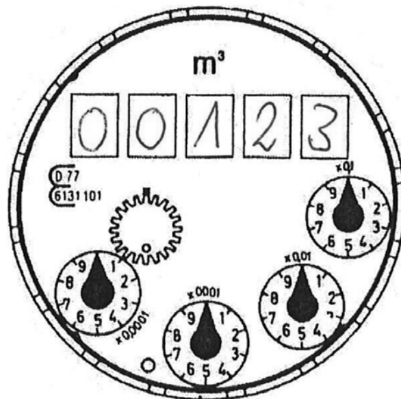
Muster eines Zählwerks eines Wasserzählers
