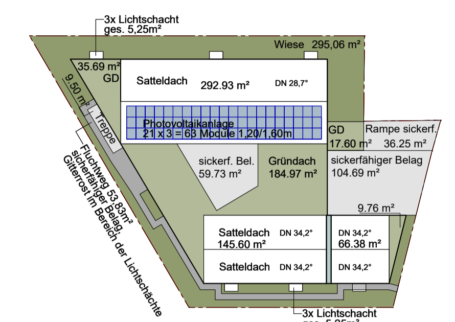
DACHAUFSICHT / BEFESTIGTE FLÄCHEN 1:500
